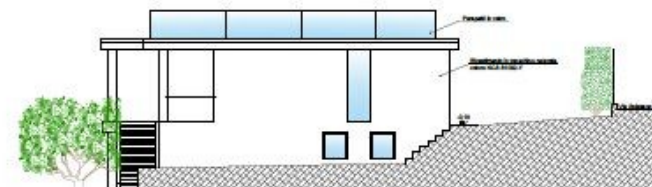
PROSPETTO EST
